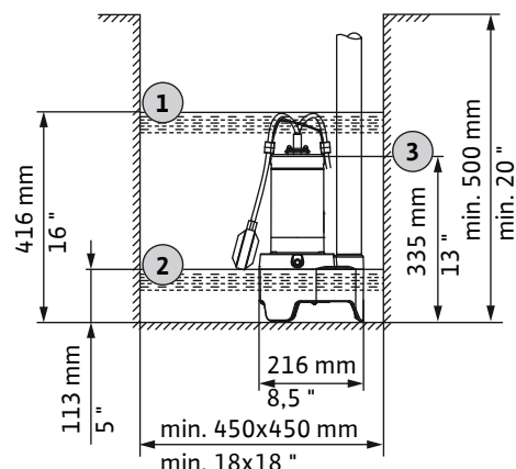
Fig. 2: Διαστάσεις εγκατάστασης και σημεία ενεργοποίησης
