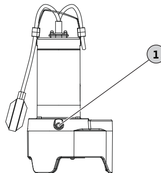
Fig. 3: Αλλαγή λαδιού θαλάμου στεγανοποίησης
